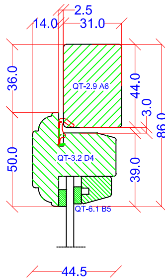
Lodrette snit
