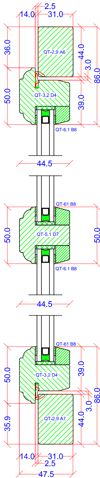
Lodrette snit
