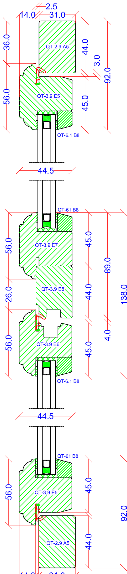
Vandrette snit
