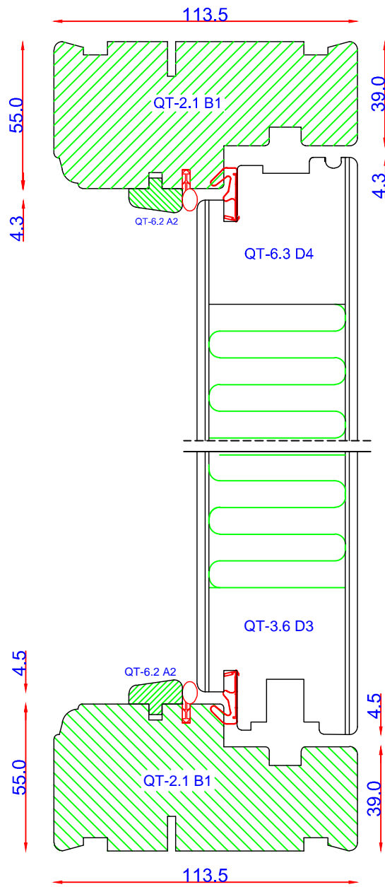
Vandrette snit
