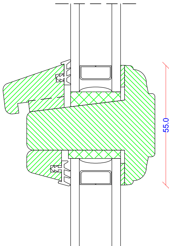
55 mm. sprosse med træ glasliste
