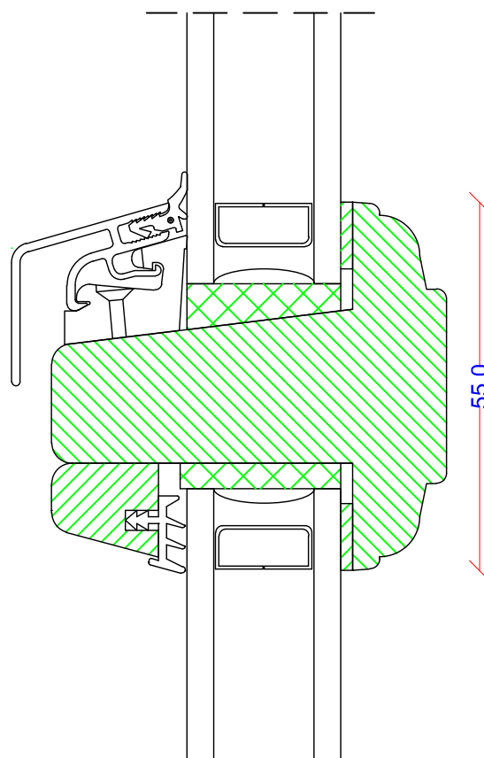
55 mm. sprosse med alu glasliste
