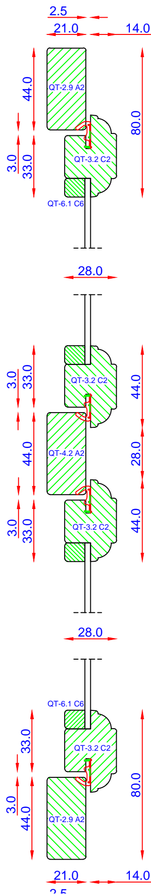
Vandrette snit
