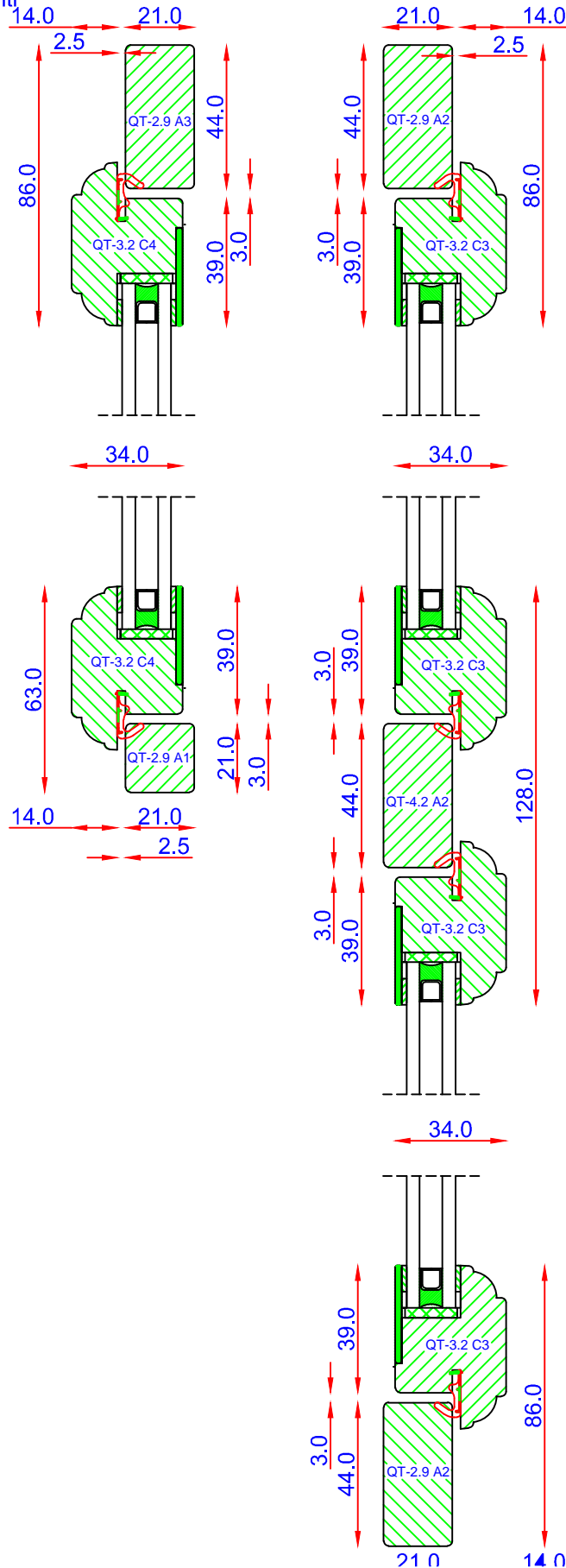
Lodrette snit
