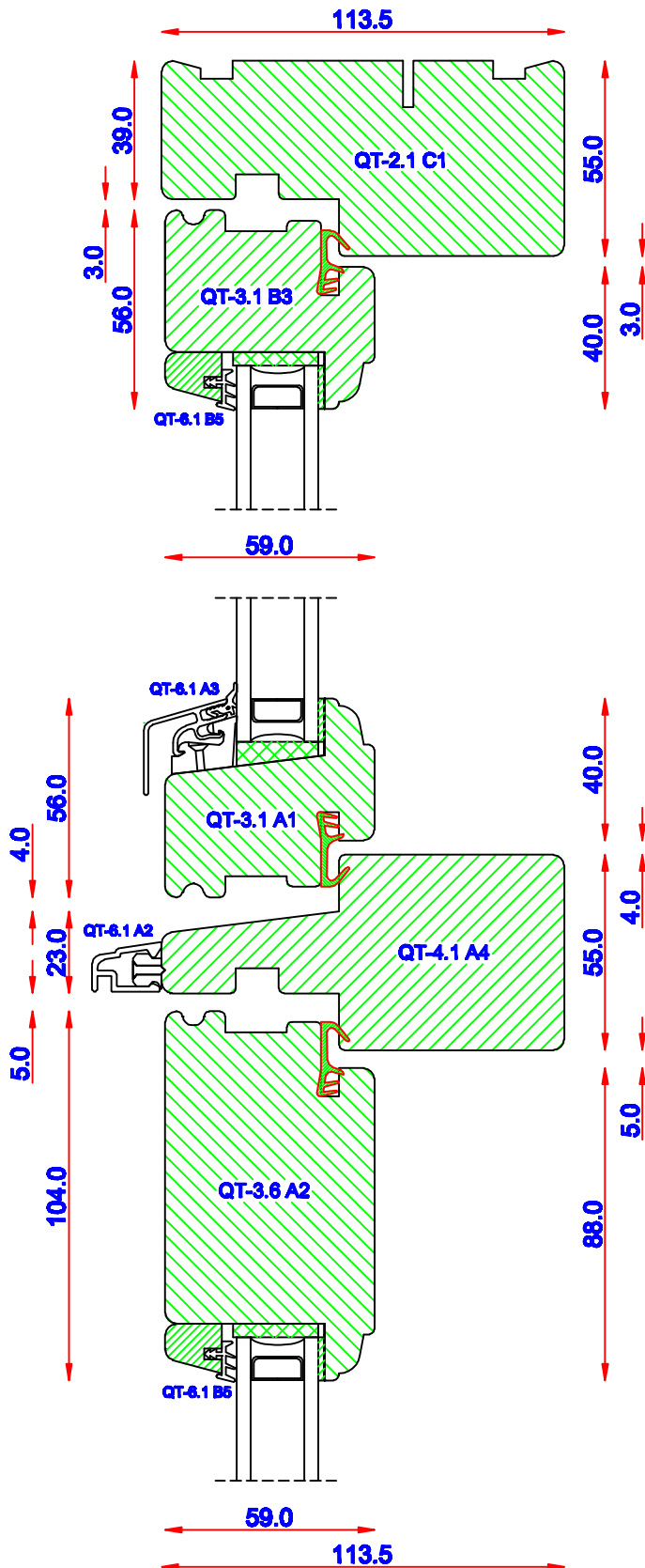
Lodrette snit
